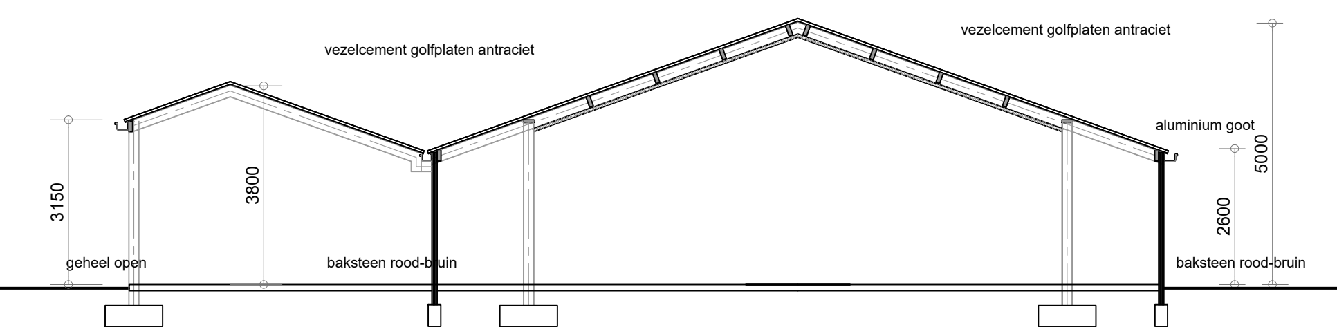
- Doorsnede A - A -
